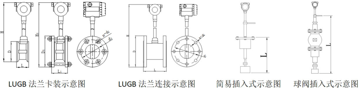
法兰卡装普通现场显示外形尺寸
