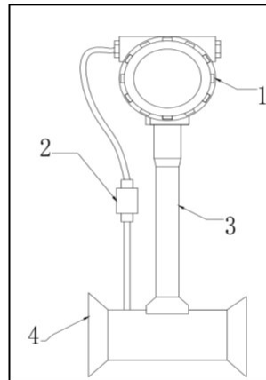
LUGB 涡街流量计产品结构图
